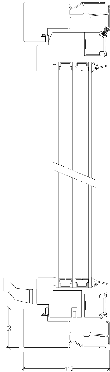
Sektion A-A
