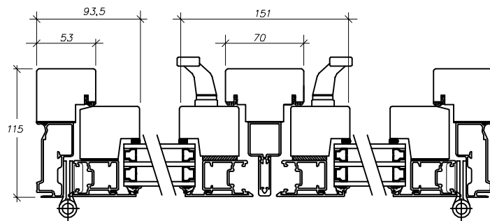
Tvåluftsfönster
