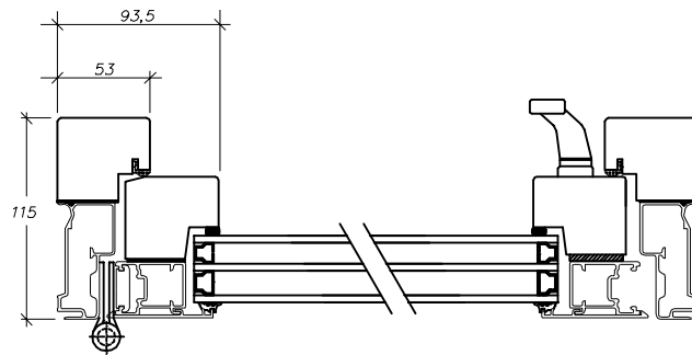
Enluftsfönster
