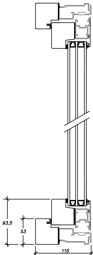
Salningsspår
