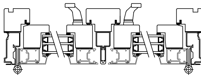
Utsida kittfalsutförande
